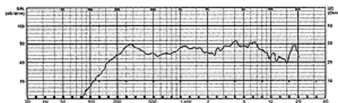
charakterystyka przenoszenia
