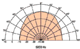
charakterystyka kierunkowa 5000 Hz
