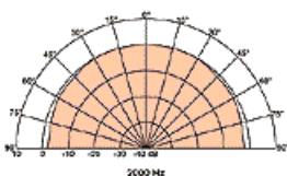
charakterystyka kierunkowa 2000 Hz
