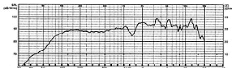
charakterystyka przenoszenia
